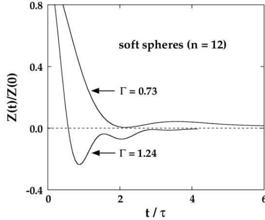
Figura 1.2: La función de autocorrelación de velocidades normalizada r^{-12} fluido en dos diferentes valores de dimensiones con parametros de acoplamiento
