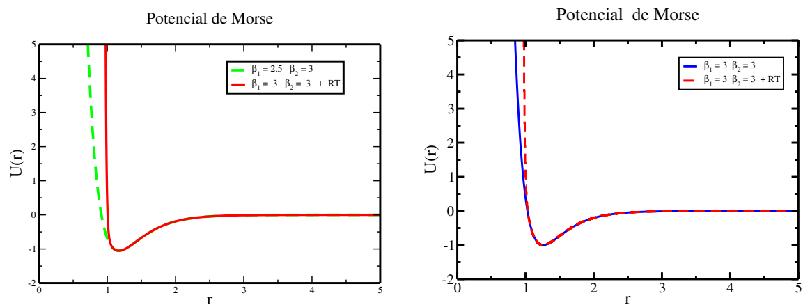
Figura 2.4: Potencial de Morse con tres repulsiones diferentes
